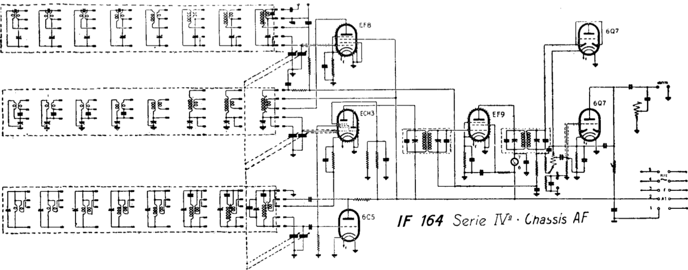
IMCARADIO. — Mod. IF164. — Quarta serie. (Nello schema è indicato solo la parte a radiofrequenza). — Produzione 1941-1942. Media frequenza: 467 kHz.
